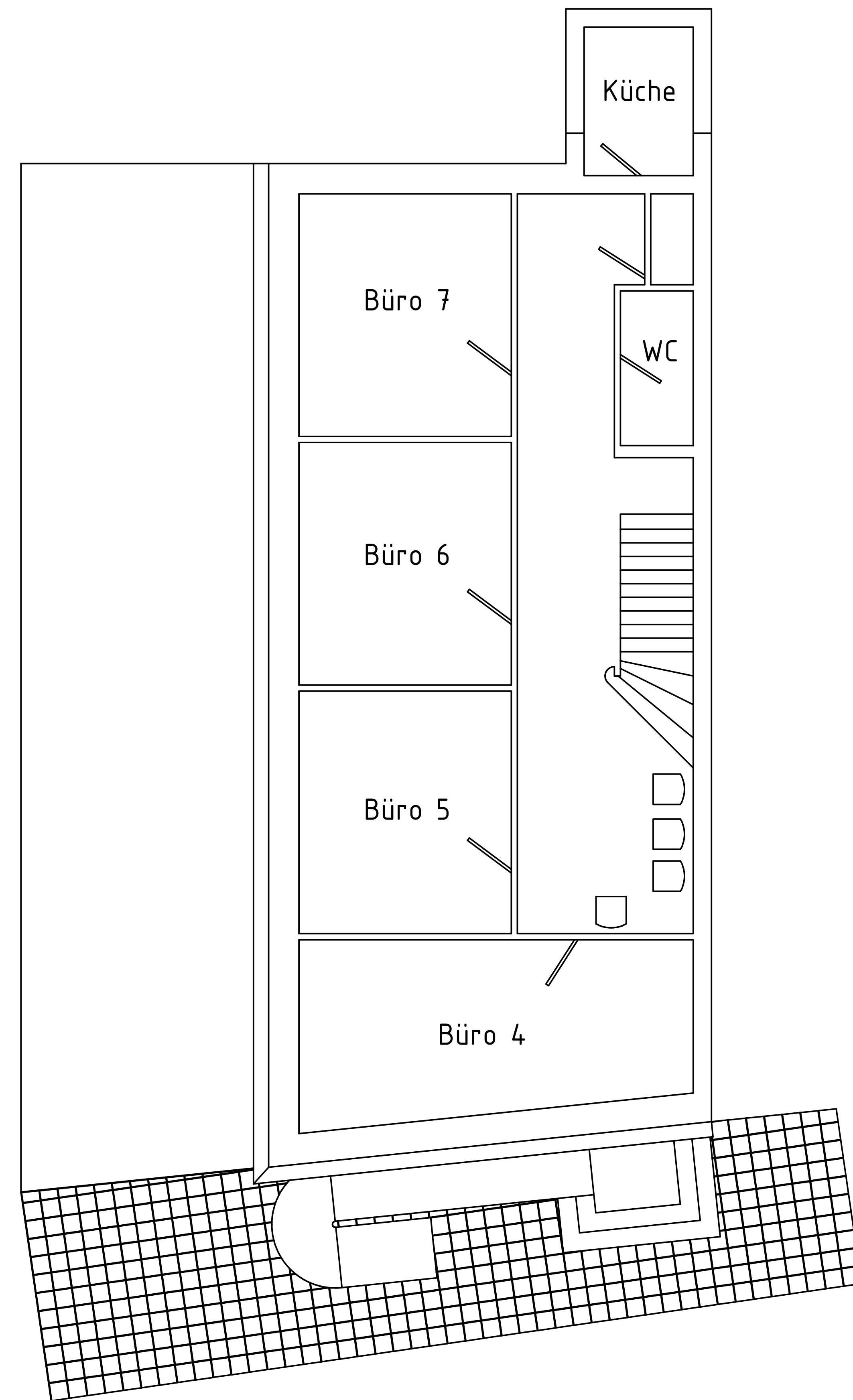
Erste Etage 1:50
