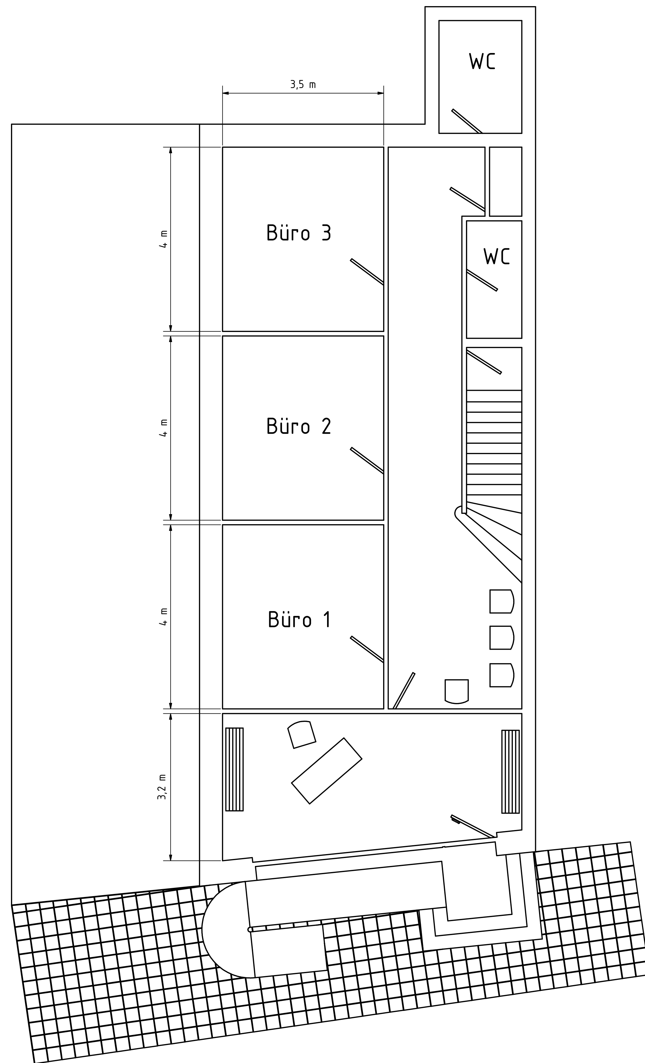
Erdgeschoss 1:50
